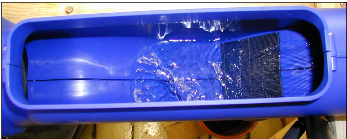
Abbildung 5: INTEWA Wechselsprungfilter WSP100 mit Q = 0,2 l/s
