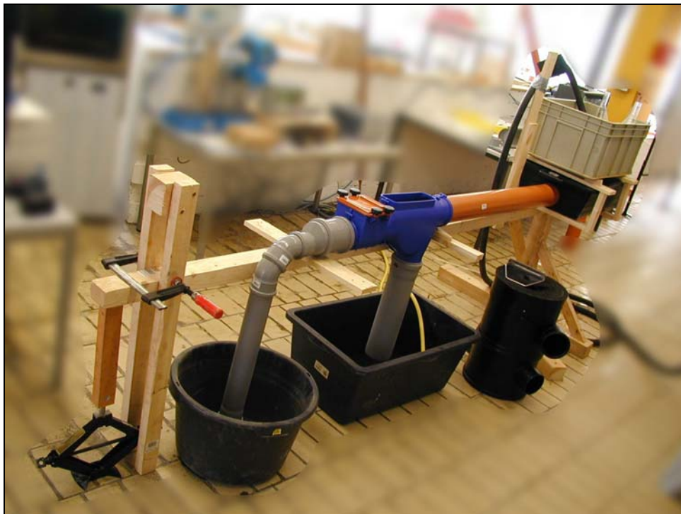
Abbildung 1: Versuchsaufbau für den Filtervergleichstest der Regenwasserfilter
