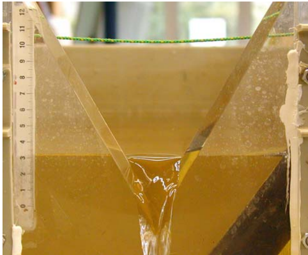
Abbildung 2: Thompsonwehr mit Q = 0,1 \text{ l/s}
