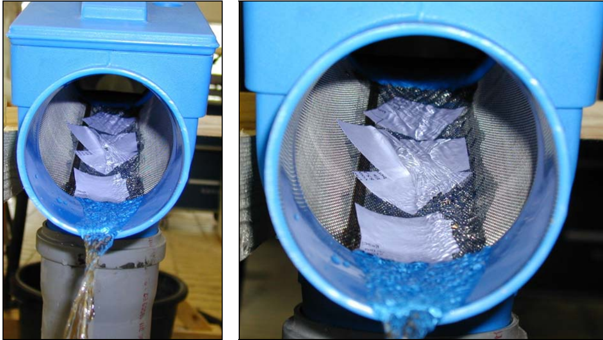
Abbildung 14: (links) 3P Patronenfilter PF mit Q = 0,2 \text{ l/s} und Verschmutzung (Papier)
