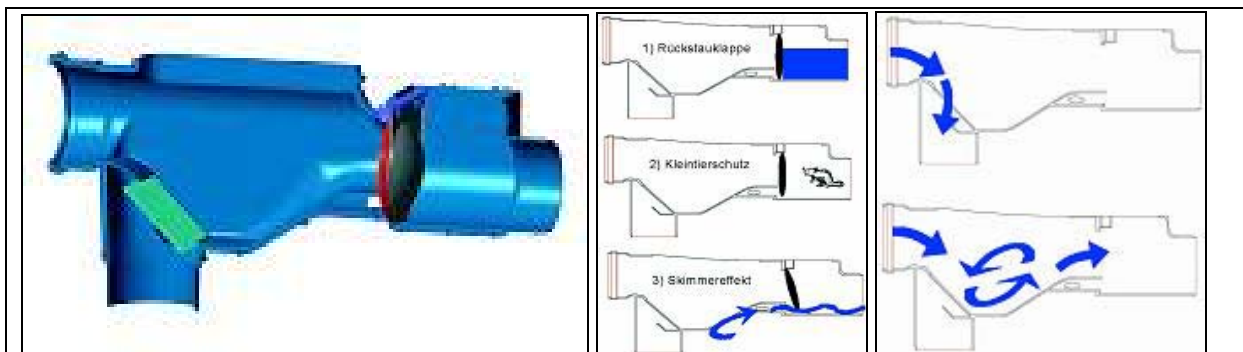
Abbildung 3: INTEWA Wechselsprungfilter WSP100
