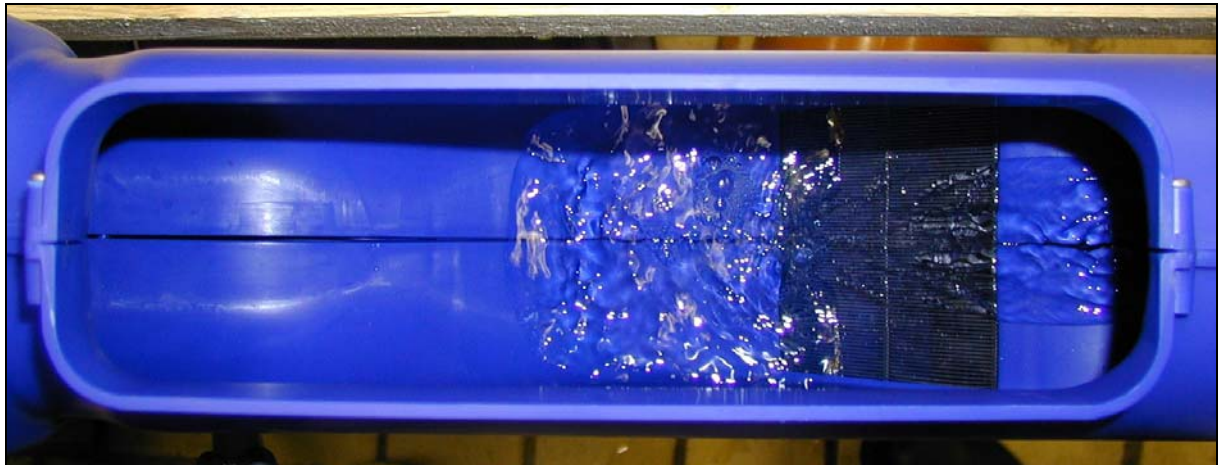
Abbildung 4: INTEWA Wechselsprungfilter WSP100 mit Q = 0,1 l/s
