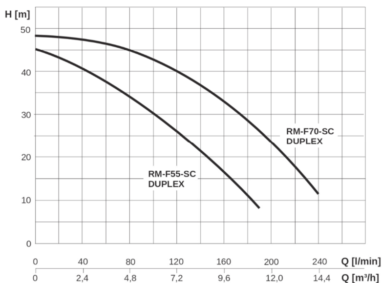
Diagr.: Druckkennlinie für RM-F55/70-SC Duplex
