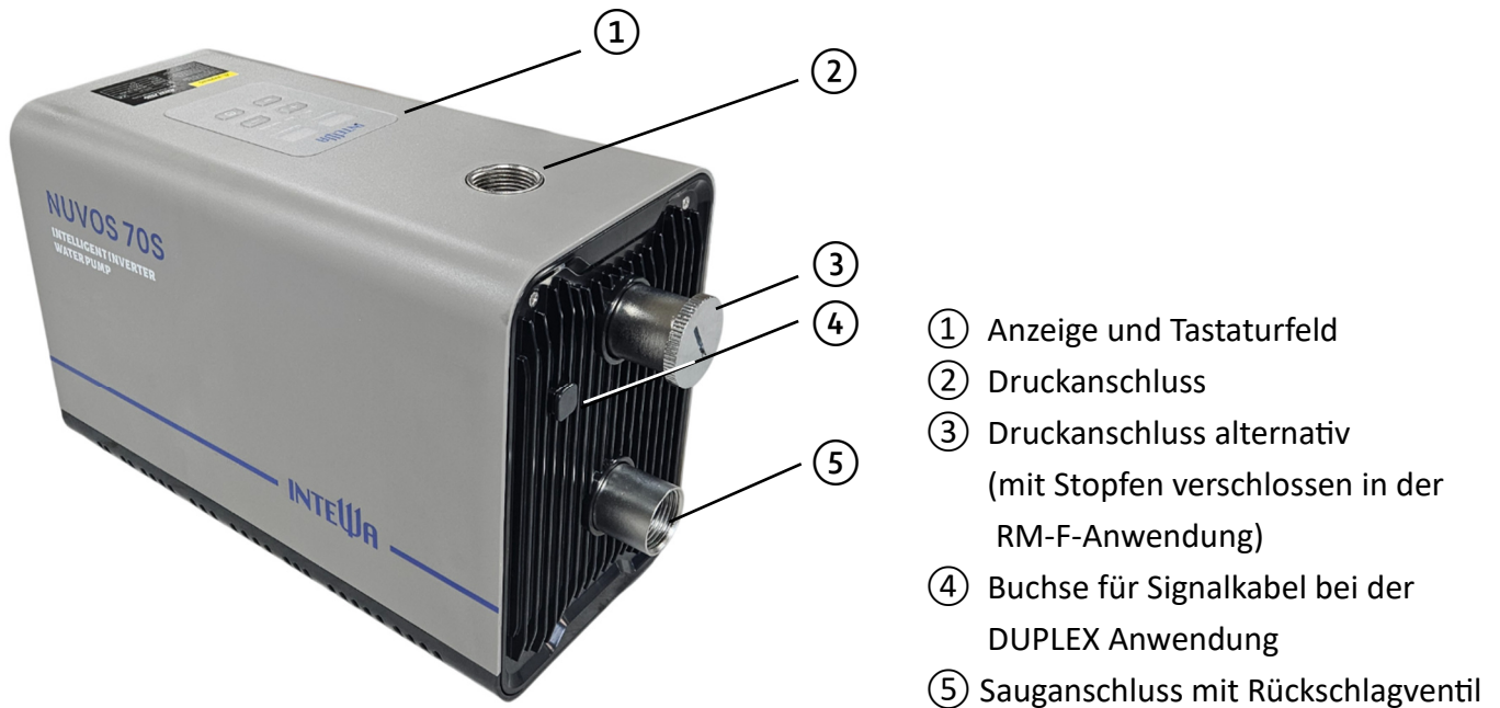
Abb.: Pumpenanschlüsse und Display
