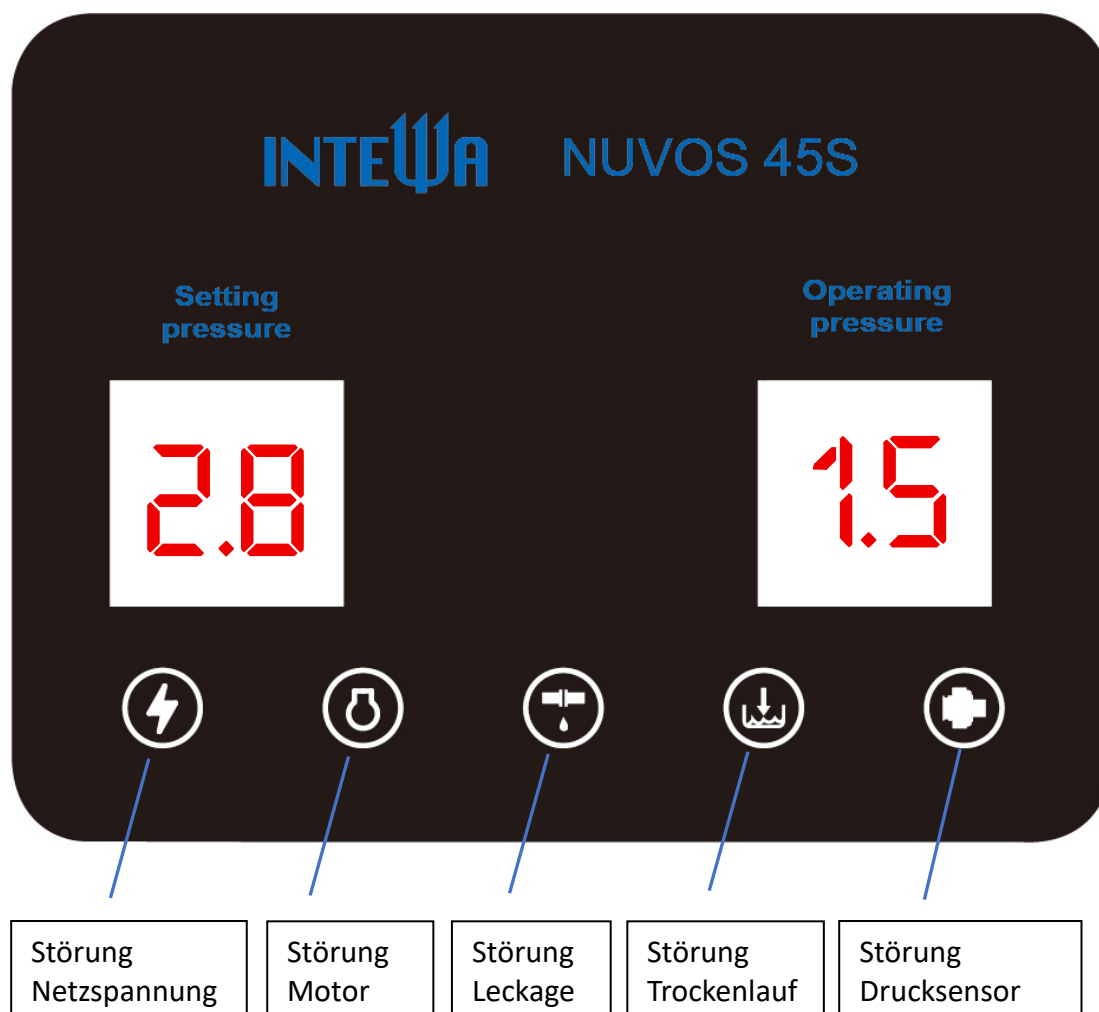
Abb.: Anzeigenfeld RM-F45-SC-A
